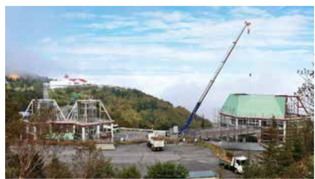
作業が進む解体工事(令和8年9月23日)
